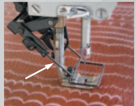
Fadenwisereinrichtung -909/93 für sauberen Nahtanfang Thread wiper mechanism -909/93 for clean seam start
